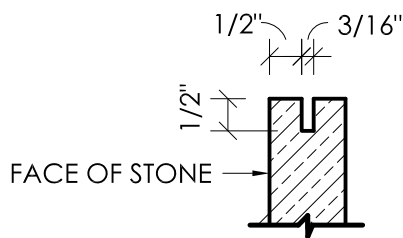
2 DETAIL - KERF SLOT
