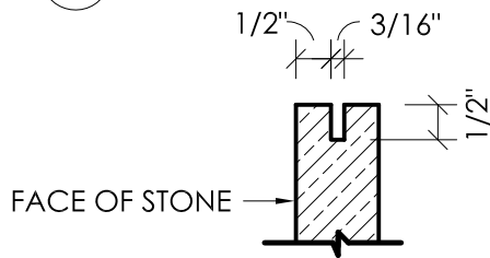
2 STONE PANEL - EDGE
