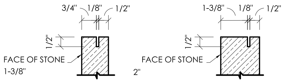
② DETAIL - KERF SLOT
