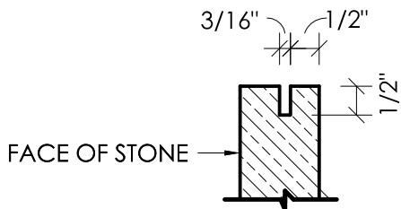
③ DETAIL - KERF SLOT
