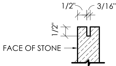
2 DETAIL - KERF SLOT
