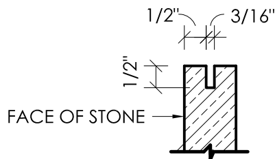
② DETAIL - KERF SLOT
