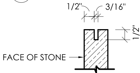
3 DETAIL - KERF SLOT
