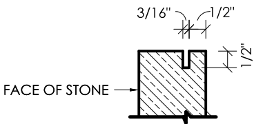
③ DETAIL - KERF SLOT
